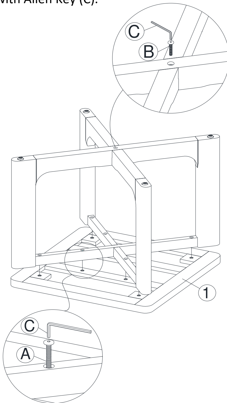
B. Bolt M6x45
